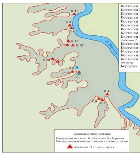
СХЕМА РАСПОЛОЖЕНИЯ СТОЯНОК В КОСТЕНКОВСКОМ РАЙОНЕ ВО ВРЕМЯ ВОРМЬСКОГО ОЛЕДЕНЕНИЯ
